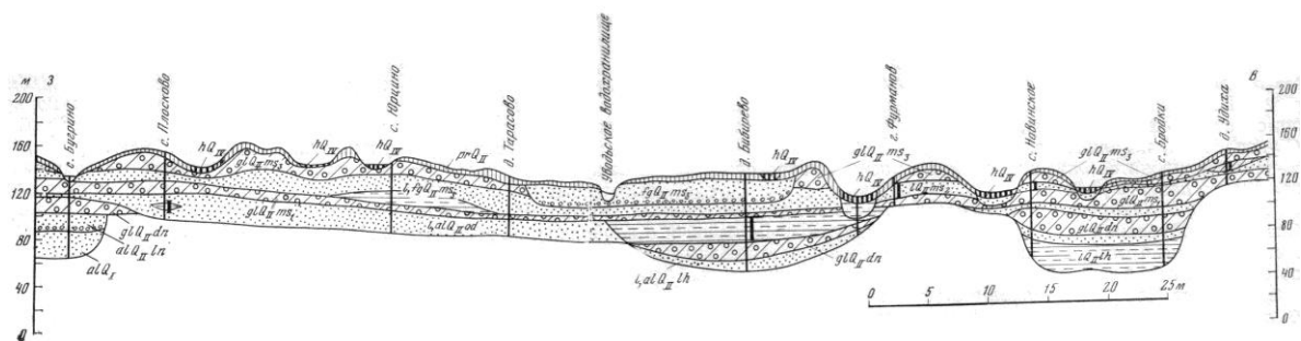
Рис. 1. Геологический профиль четвертичных отложений северной г. Иваново, по данным С.М. Шика
